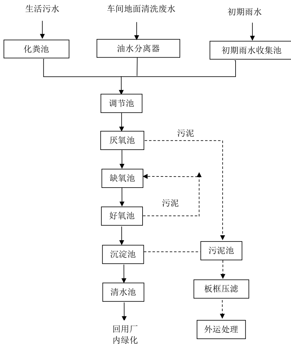
图 7 本项目污水处理设施工艺流程图
